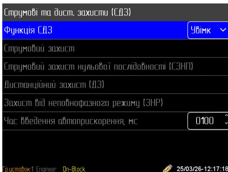
Рисунок 5.5.3.1 – Меню налаштувань функцій СДЗ
