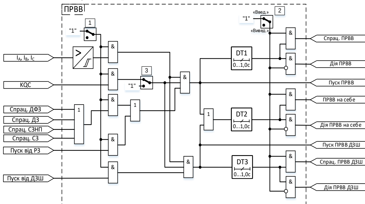
Рисунок 4.2.1 – Схема ПРВВ
