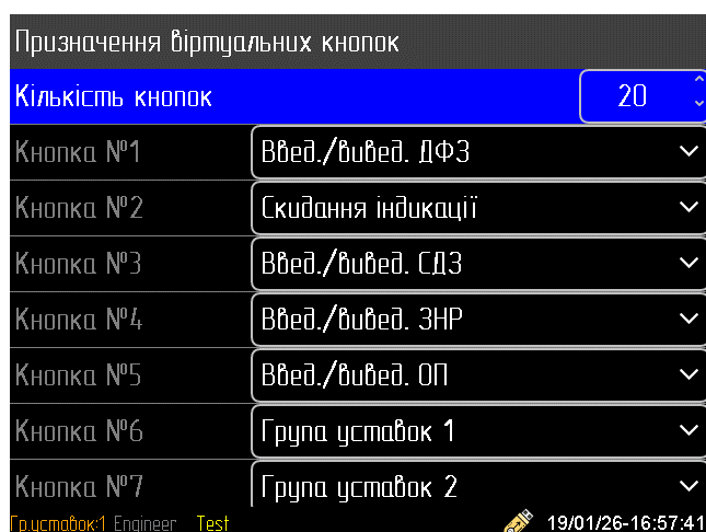
Рисунок 5.4.9.2. Меню налаштувань «Віртуальні кнопки»
