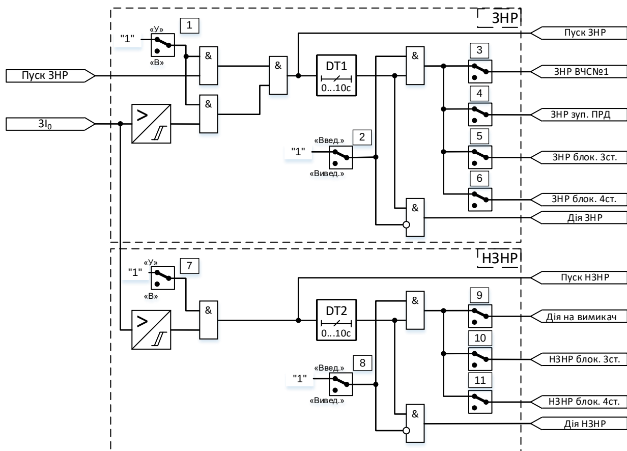
Рисунок 4.3.1 – Схема ЗНР та НЗНР
