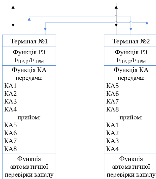
Рисунок 4.4.2 - ВЧ канал с двома терміналами «ОРИОН» ДФЗ
