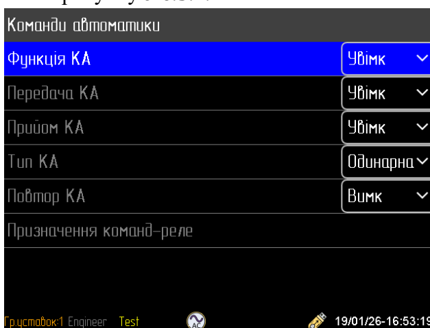
Рисунок 5.6.3.1 – Налаштування прийому та передачі команд автоматики
