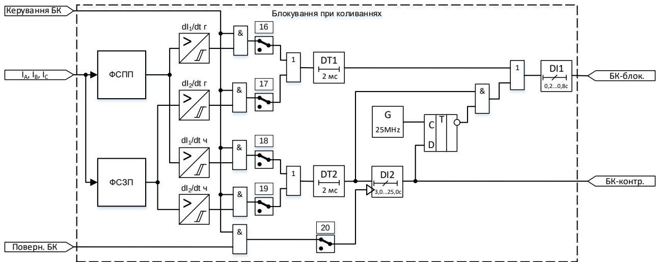
Рисунок 4.1.2.3 Схема БК
