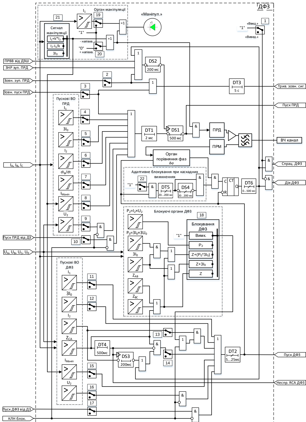
Рисунок 4.1.1.3 Схема ДФЗ
