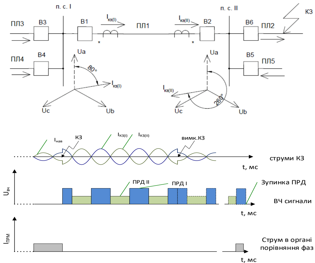
Рисунок 4.1.1.1 - КЗ на суміжній ПЛ – зовнішнє (за межами зони) для захисту ПЛ №1 Сигнал обміну ПРД маніпулюється сигналом 50 Гц з фазою струму КЗ в місці встановлення комплекту захисту. В якості сигналу маніпуляції, а також для пускових органів
