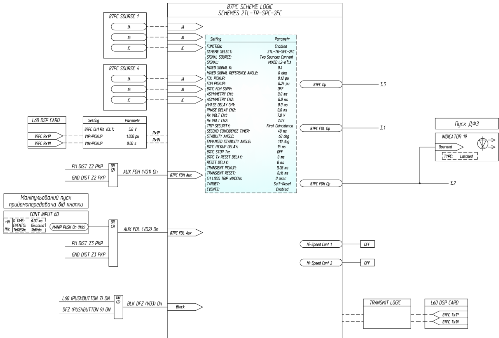
Рисунок Д3.2. – Конфігурація внутрішньої логіки L60 General Electric при сумісному використанні з ОΡΙΟΝ ДФЗ (початок)
