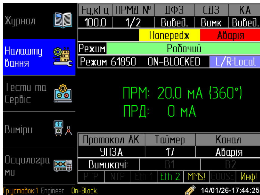
Рисунок 5.2.1 – Головний екран
