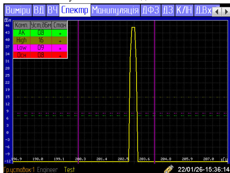
Рисунок 5.9.4 – Вкладка «Спектр».
