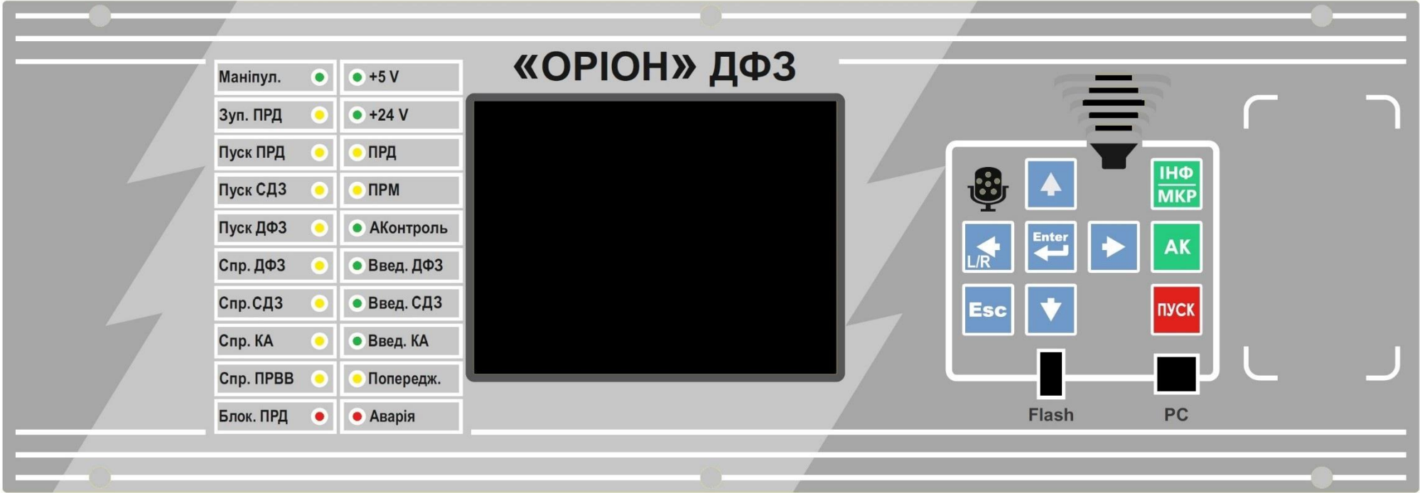
Рисунок 6.3 – Зовнішній вигляд лицьової панелі «ОРИОН» ДФЗ (виробництво до 01.10.2025)
