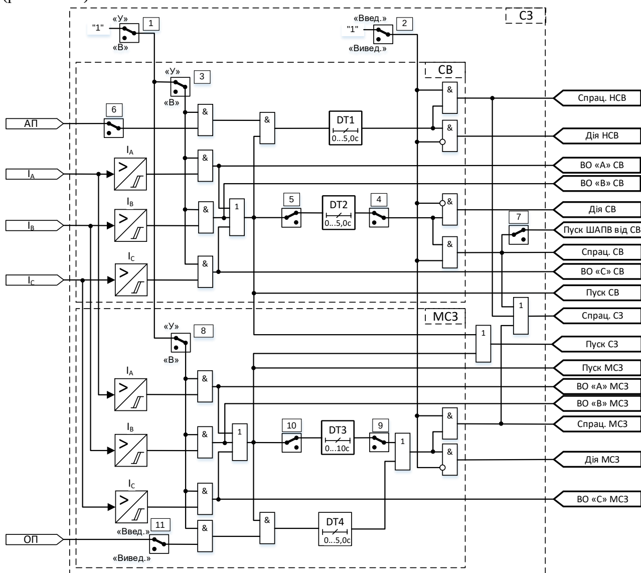
Рис. 4.1.4.1 Схема СЗ
