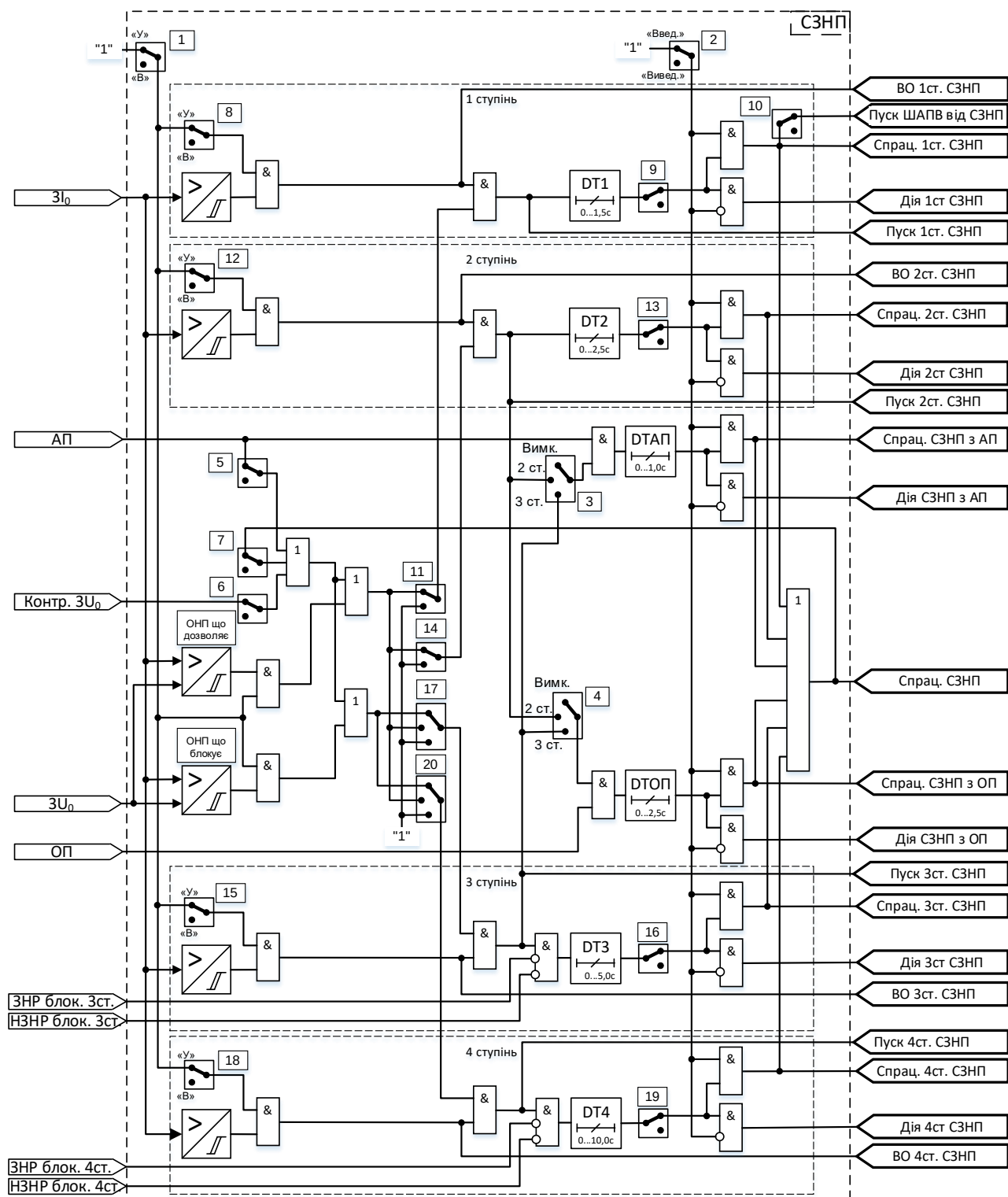
Рисунок 4.1.3.1 Схема СЗНП
