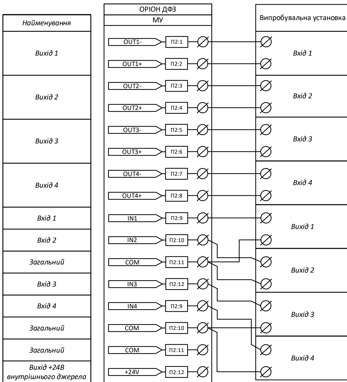
Рисунок Д1.6.2 - Схема підключення налагоджувально-випробувального модуля в МУ до перевірконої установки (РЗА Тестер, OMICRON CMC356)
