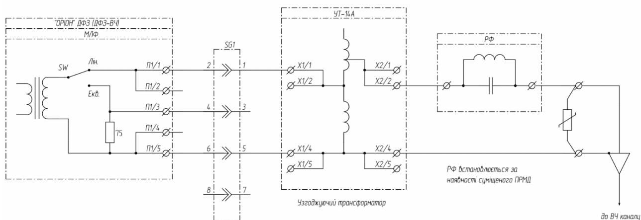
Рисунок Д1.7.1 - Схема підключення до ВЧ каналу
