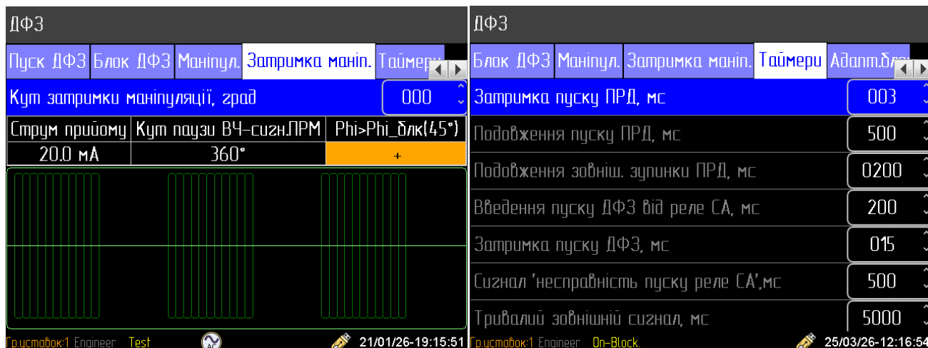
Рисунок 5.5.2.1 – Налаштування диференційно-фазного захисту
