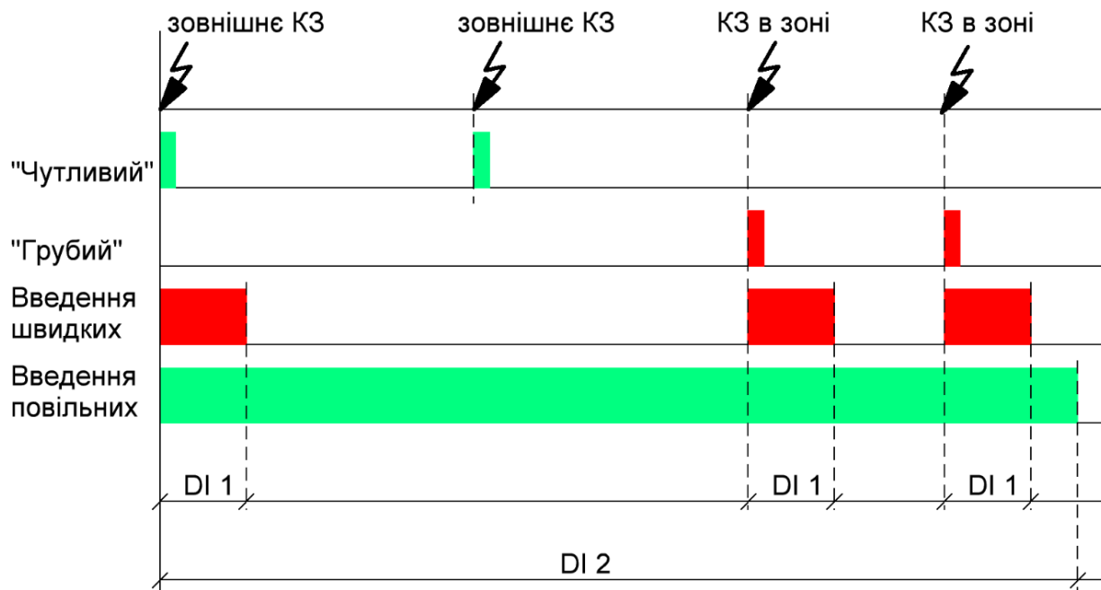
Рисунок 4.1.2.4 Діаграма роботи БК
