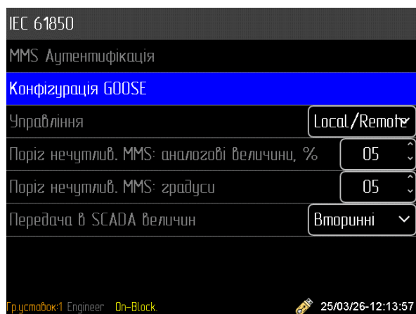
Рисунок 5.4.5.1 – Меню «IEC 61850»
