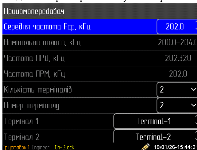
Рисунок 5.6.1.1 – Налаштування прийомопередавача
