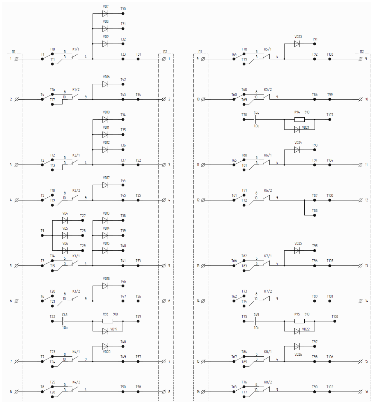
Рисунок Д1.4.2 – Схема вихідних ланцюгів МУРС2
