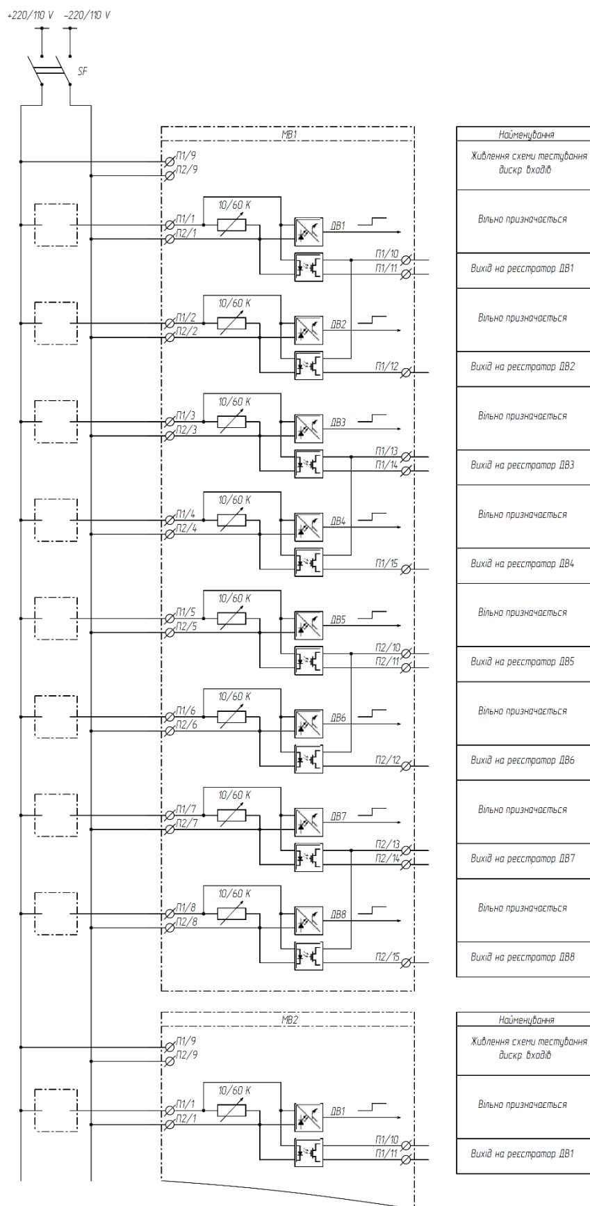
Рисунок Д1.2.1 – Підключення MB1, 2
