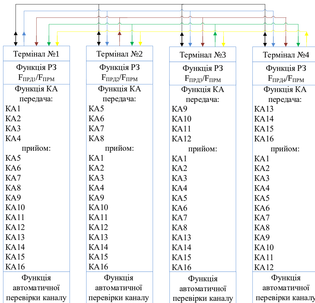
Рисунок 4.4.4 - ВЧ канал с чотирма терміналами «ОΡΙΟΝ» ДФЗ
