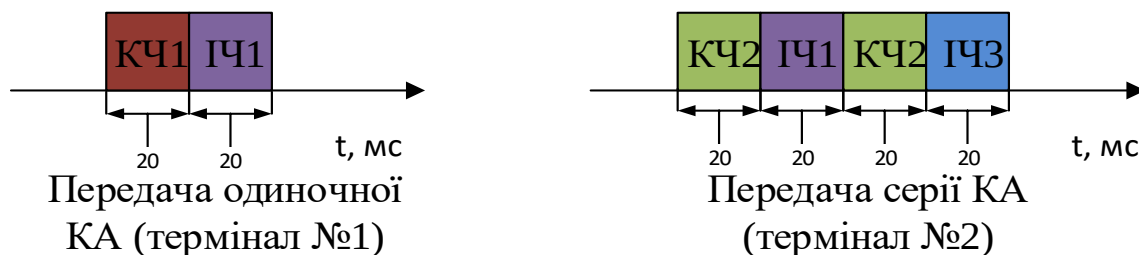
Рисунок 4.4.1 - Передача команд автоматики
