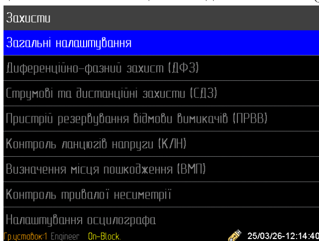
Рисунок 5.5.1. – Загальний вигляд розділів меню «Налаштування захистів»
