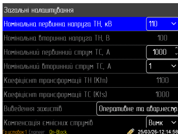
Рисунок 5.5.1.1 – Загальні налаштування
