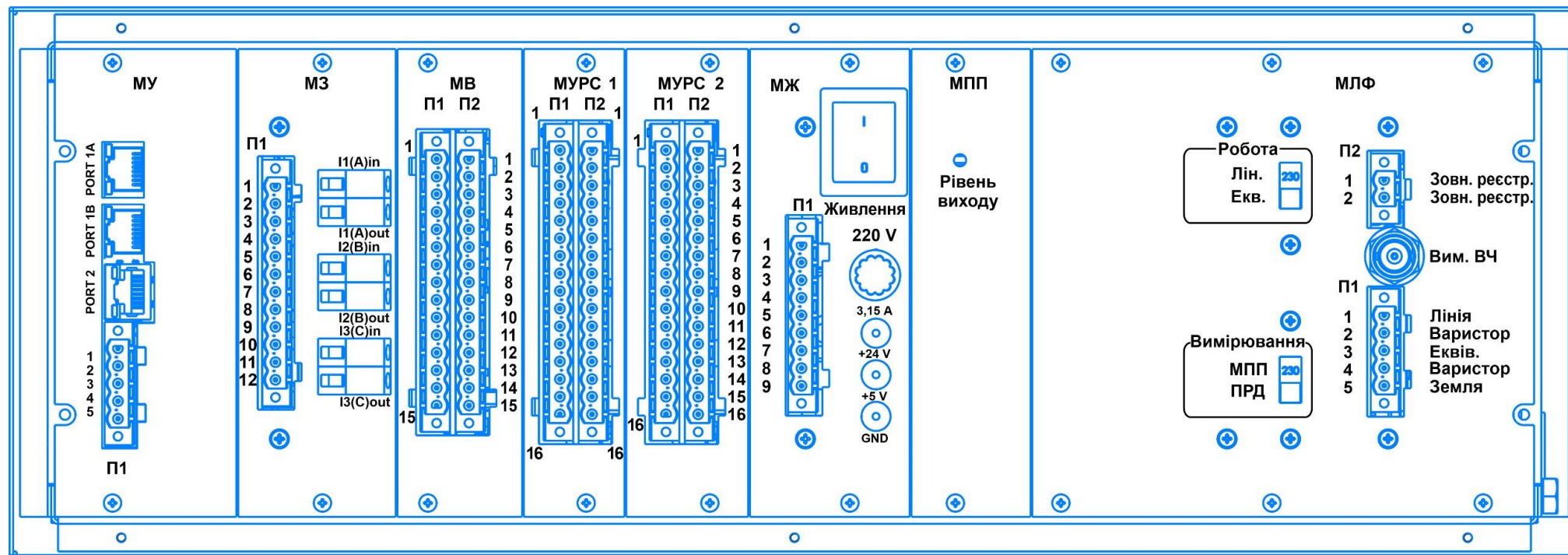
Рисунок 6.5 – Зовнішній вигляд «ОРІОН» ДФЗ зі сторони підключення (виробництво до 01.10.2025)
