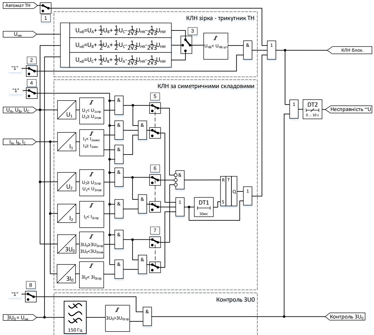
Рисунок 4.8.1 – Схема контролю ланцюгів напруги
