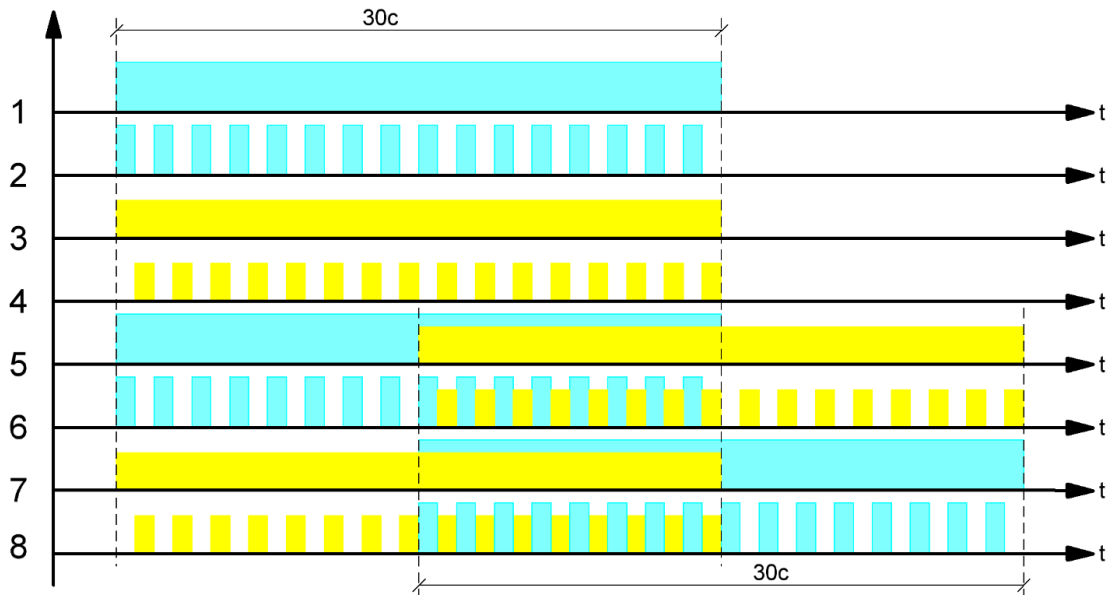
Рисунок 4.6.1 – Можливі ситуації у каналі зв'язку при оперативному пуску та дистанційному відгуку:
