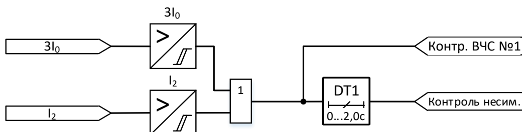
Рисунок 4.9.1. – Схема контролю тривалої несиметричності струмів
