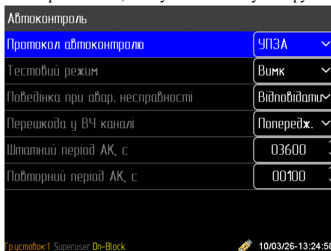
Рисунок 5.6.2.1 – Автоконтроль
