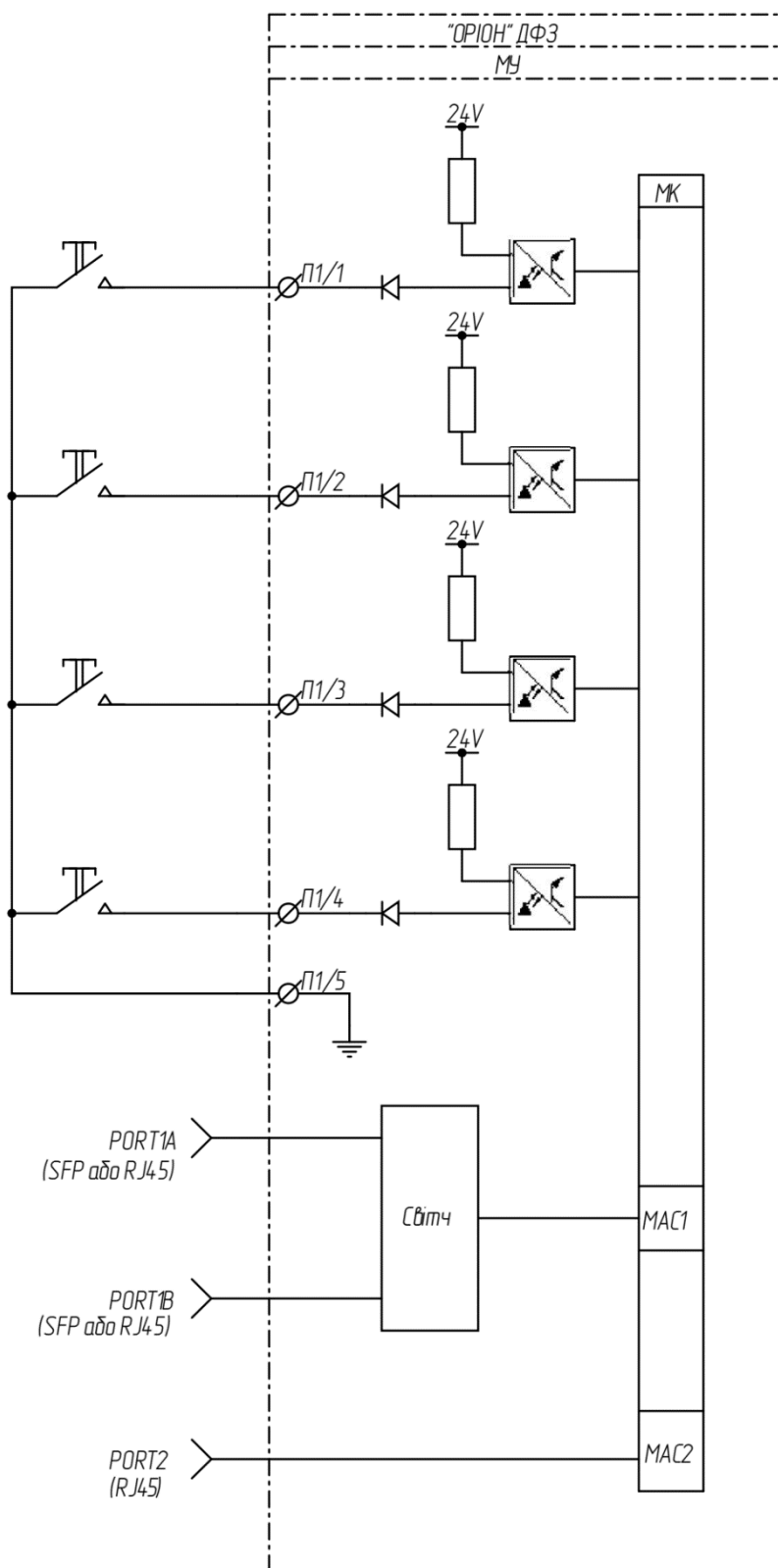
Рисунок Д1.6.1 - Схема підключення зовнішніх кнопок до МУ
