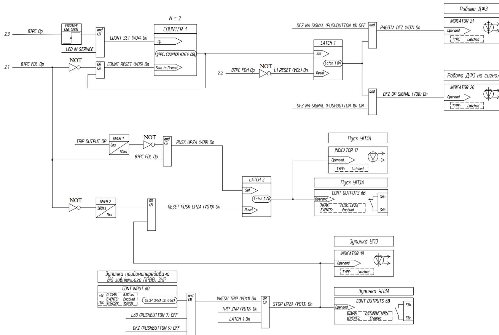
Рисунок Д3.2. – Конфігурація внутрішньої логіки L60 General Electric при сумісному використанні з ОΡΙΟΝ ДФЗ (закінчення)
