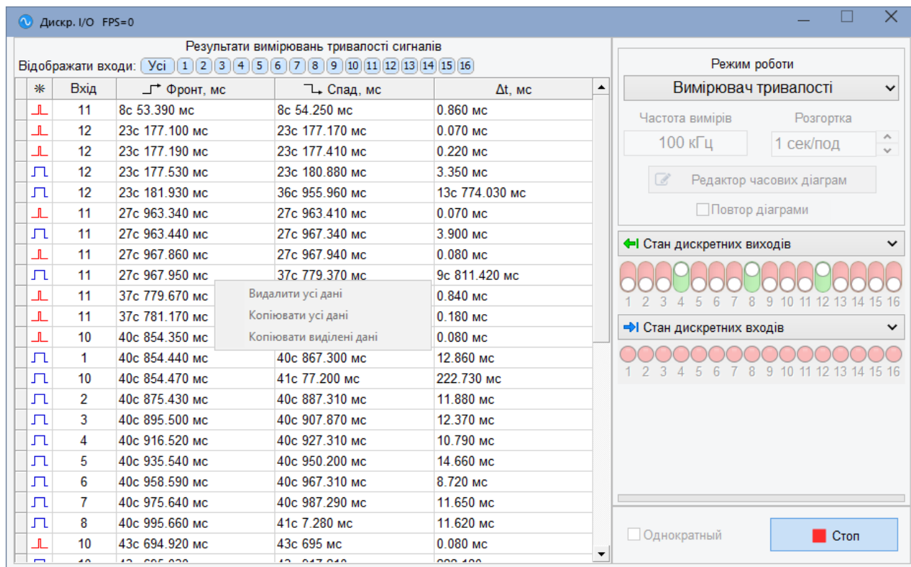
Рисунок 10.11.3.1 – Зовнішній вигляд панелі «Дискр. I/O» в режимі роботи «Вимірювач тривалості»
