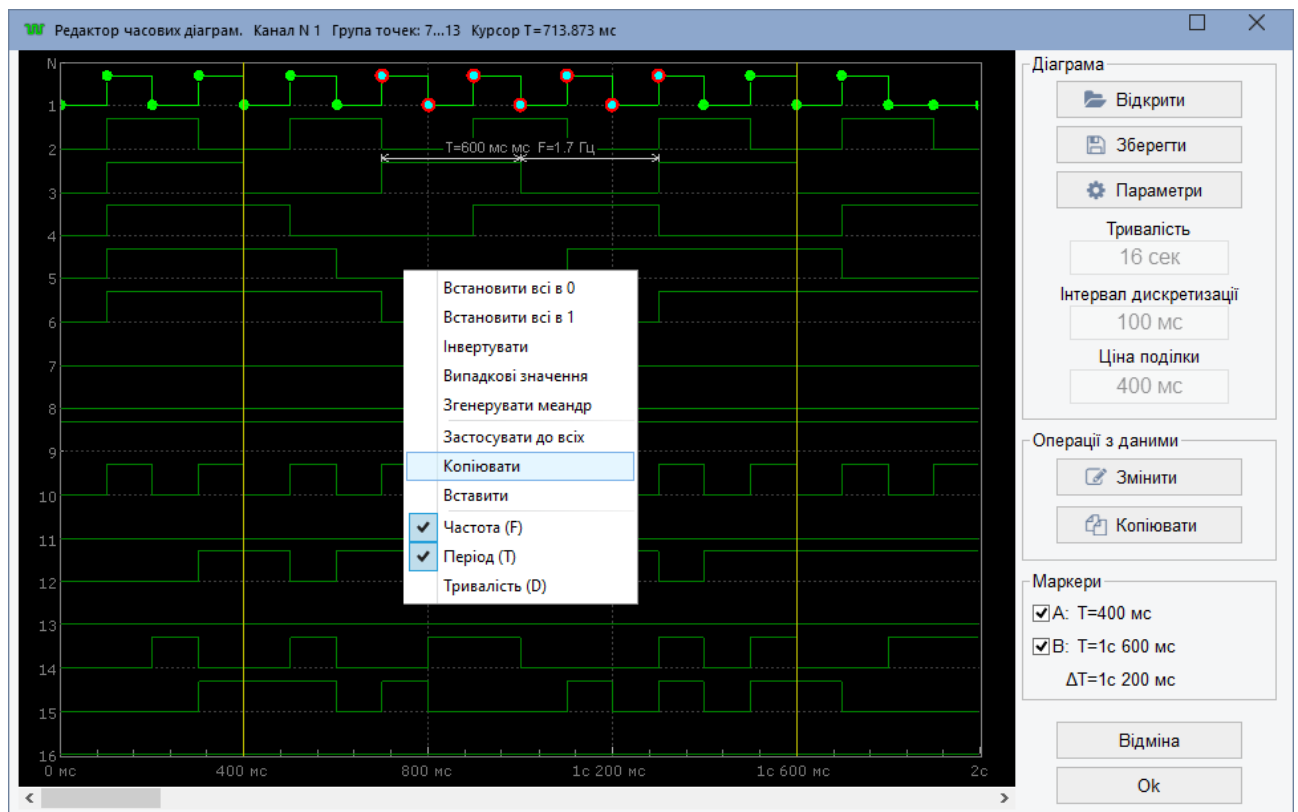
Рисунок 10.11.4.1 – Зовнішній вигляд вікна модуля «Редактор тимчасових діаграм»
