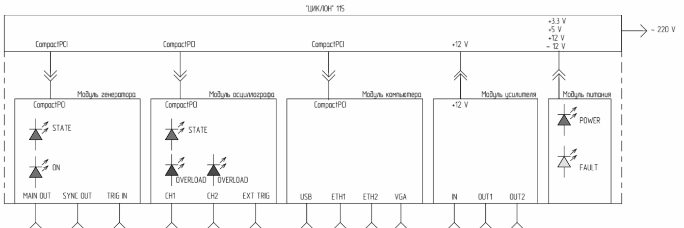
Рисунок 6.1.1 – Структура приладу
