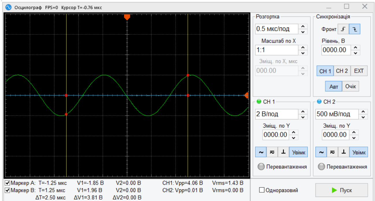
Рисунок 10.2.2.1 – Зовнішній вигляд панелі осцилографа
